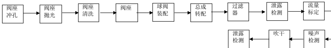
图 FBRV调压器生产线工艺流程简图
