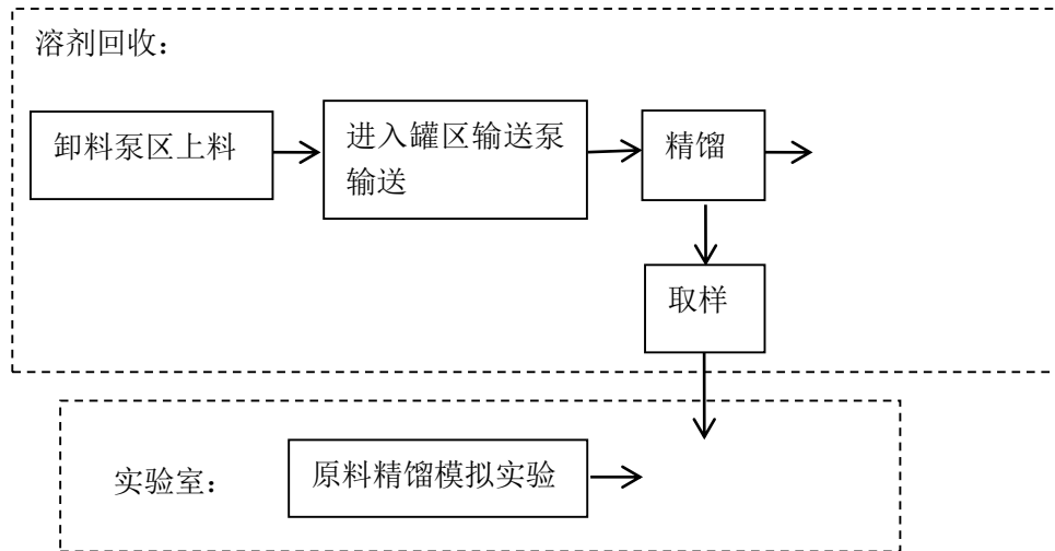
项目主要工艺流程图
