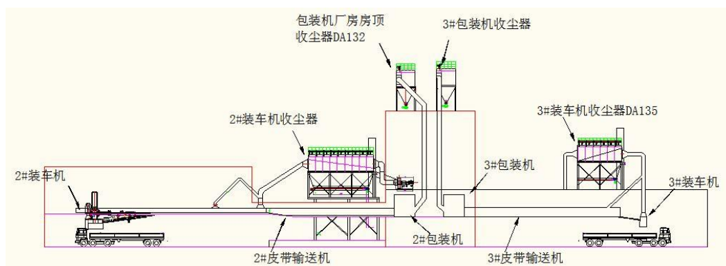
项目改造后工艺
