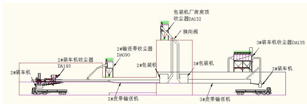
项目改造前工艺
