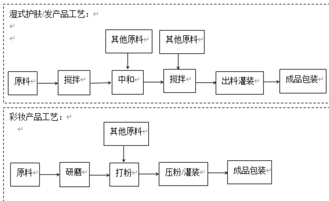
项目主要工艺流程图
