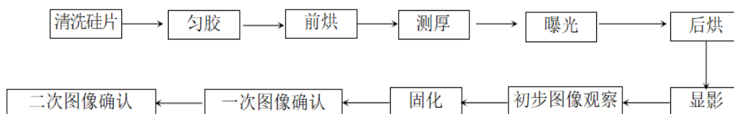
光刻工艺流程图
