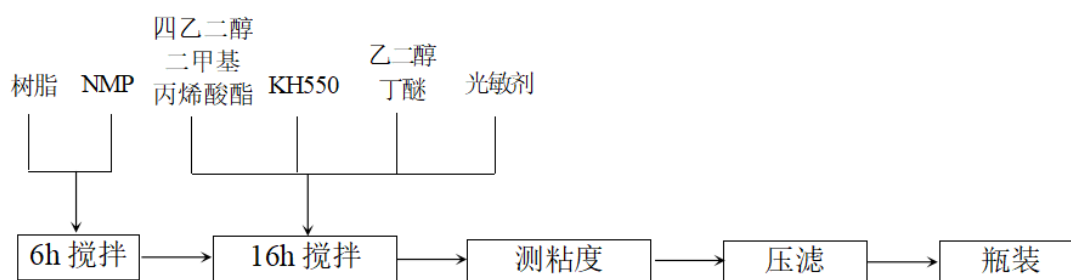
配胶工艺流程图
