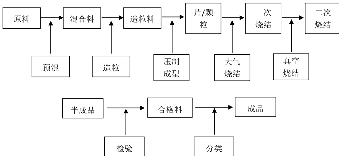
图 1 项目主要工艺流程图
